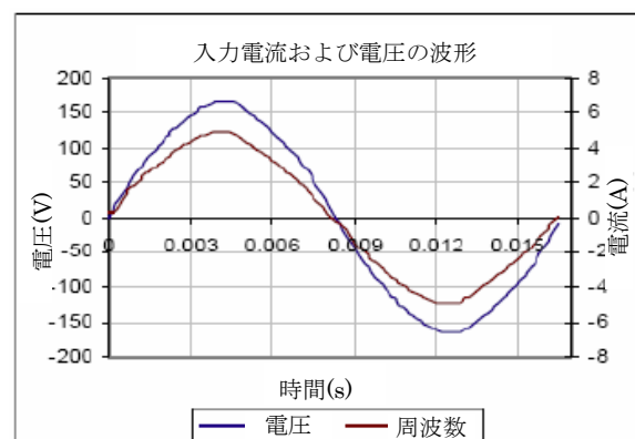
入力交流電流波形 (100% 負荷において I_{THD}=4.1\% )
